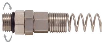
RACCORDO GIREVOLE FILETTO MASCHIO PER TUBO GOMMA E POLIURETANO TENUTA CON OR ROTATING JOINT "MALE" WITH SPRING FOR RILSAN AND POLYURETHANE HOSE WITH OR
